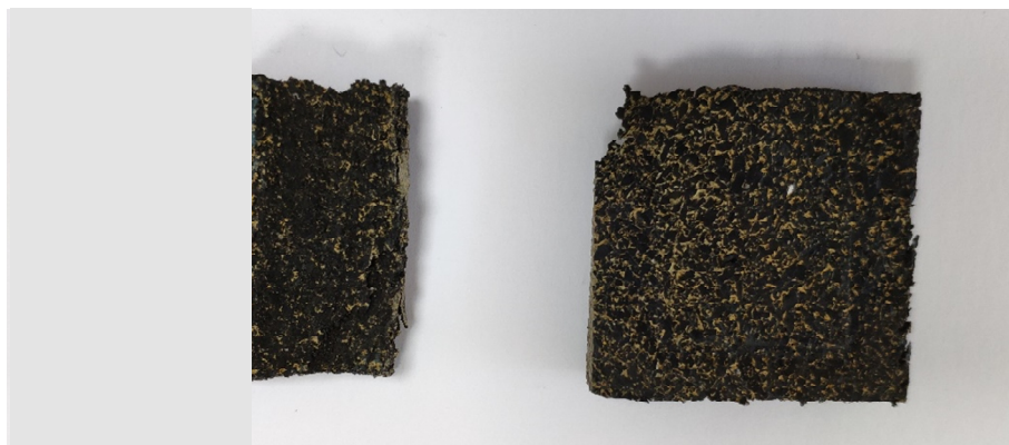
FIGURA 4. MUESTRA REF. "LOSETA NEGRA", IZQ.) SIN ENVEJECER, DER.) TRAS 1500 HORAS DE ENSAYO
