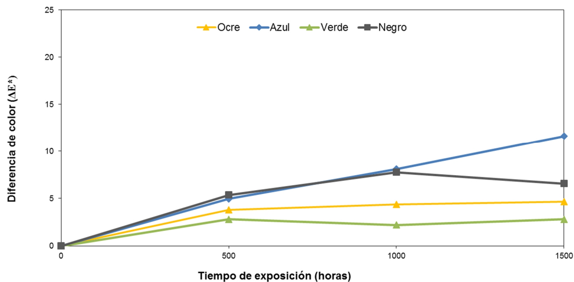
FIGURA 5. VARIACIÓN DE LA MEDIDA DE LA DIFERENCIA DE COLOR CON EL TIEMPO DE EXPOSICIÓN DE LAS MUESTRAS
