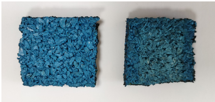
FIGURA 2. MUESTRA REF. "LOSETA AZUL", IZQ.) SIN ENVEJECER, DER.) TRAS 1500 HORAS DE ENSAYO
